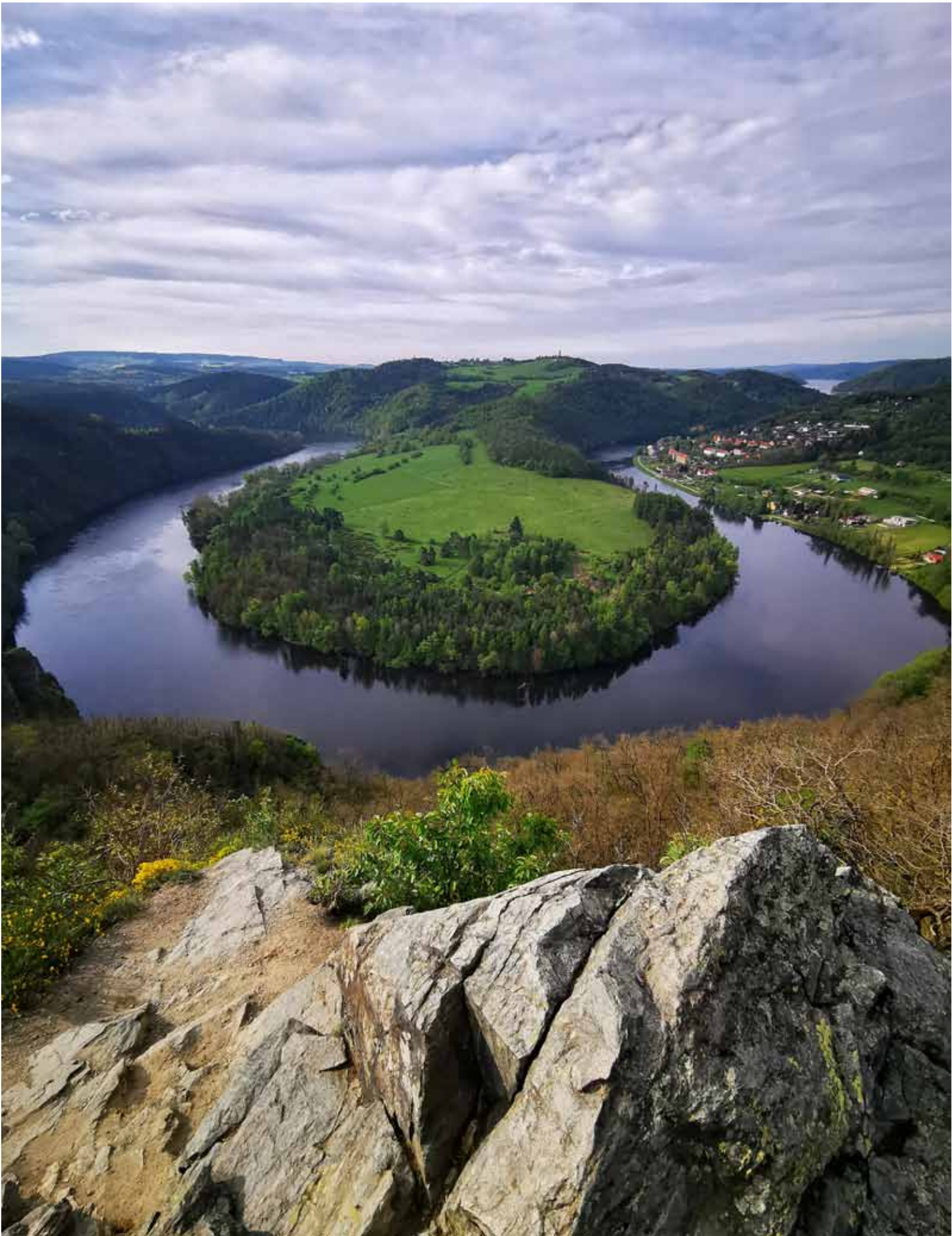
Solenická podkova
